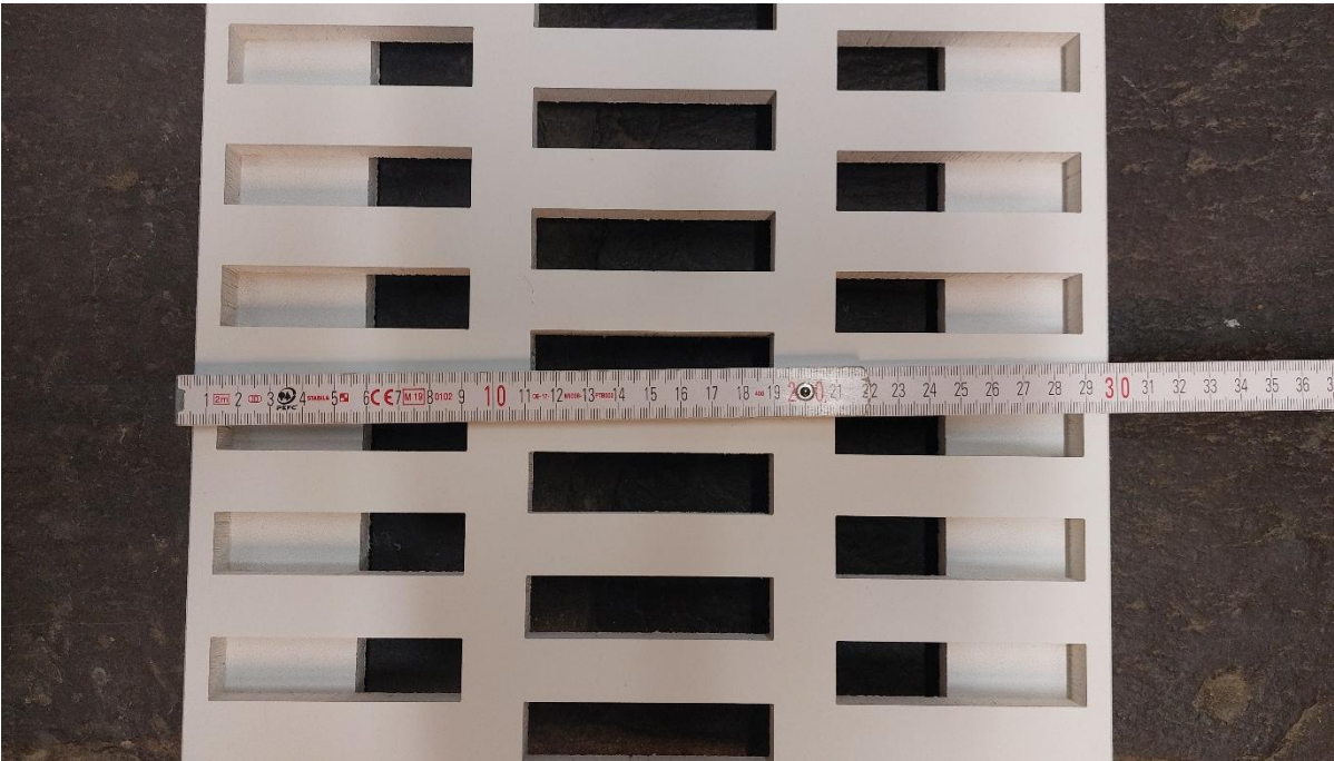
Foto 5 Quervermessung Lochung
