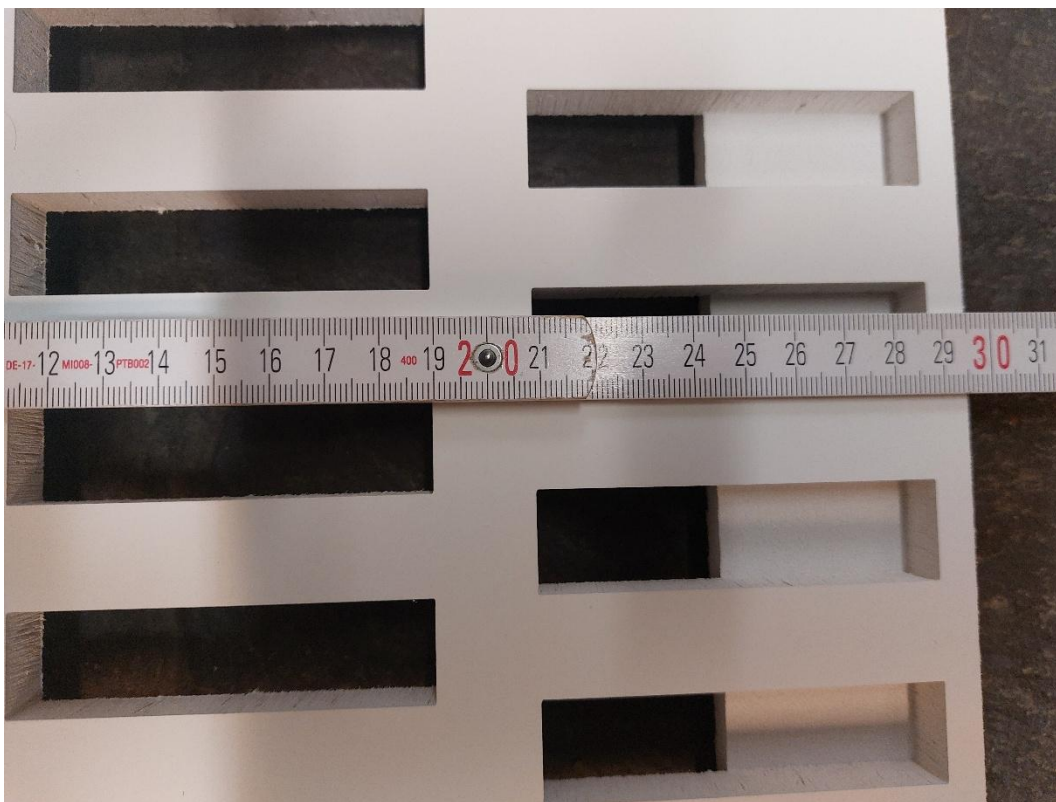
Foto 7 Quervermessung Lochung
